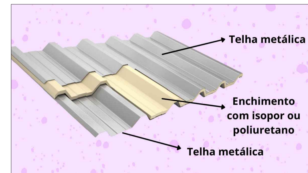
DETALHE TELHA TRAPEZOIDAL TIPO SANDUÍCHE (3 CAMADAS)
