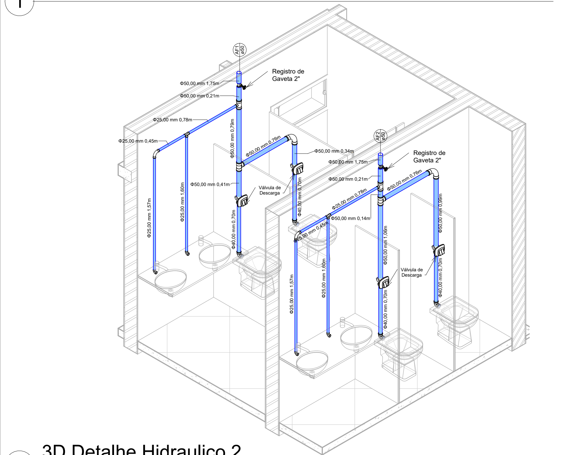
2 3D Detalhe Hidraulico 2
