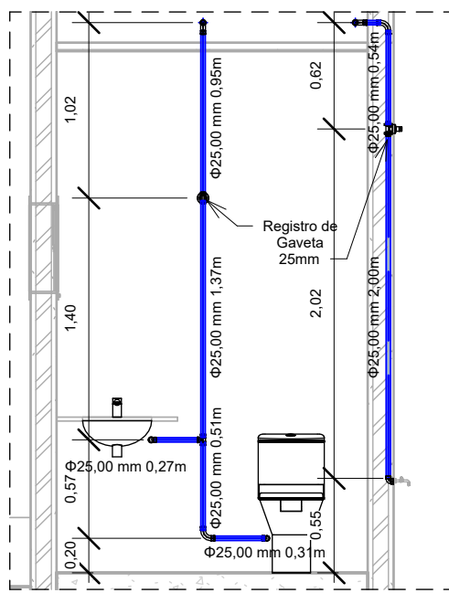
10 Detalhe 6 1 : 40
