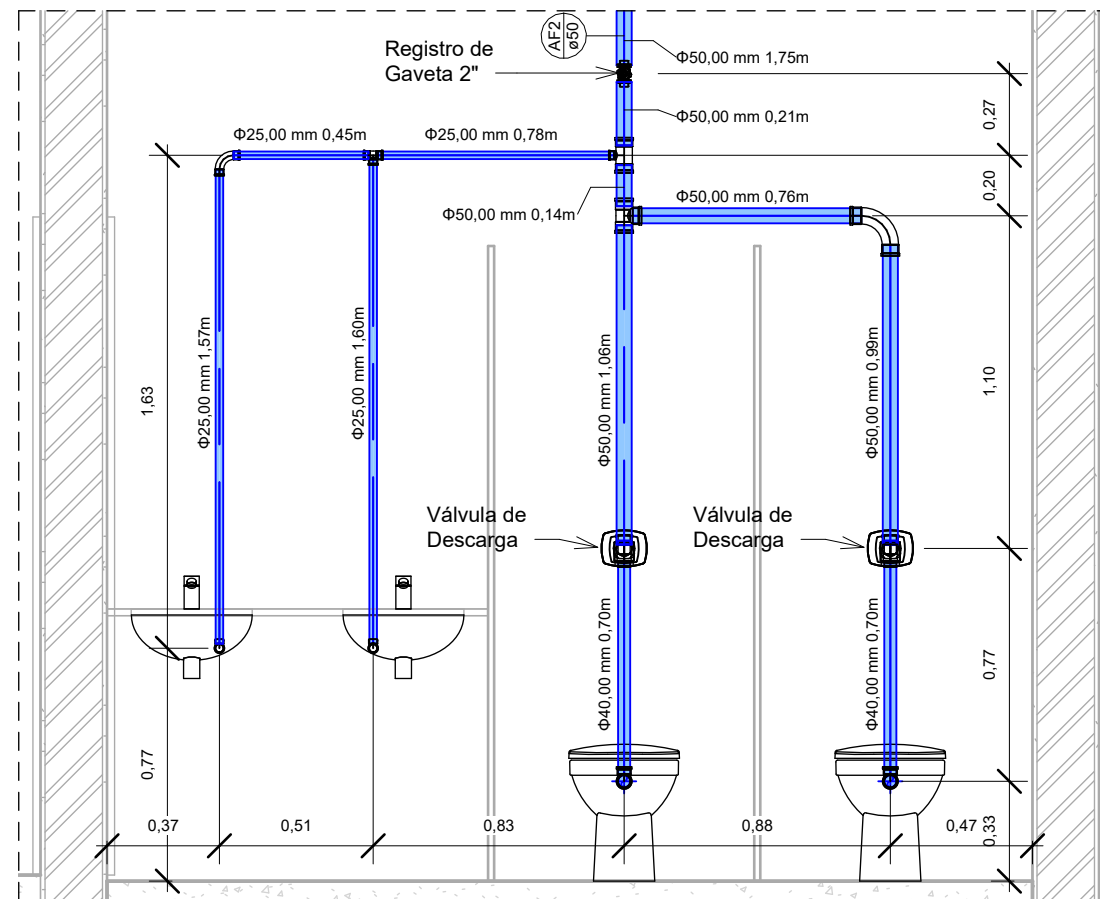
4 AF2 1 : 25
