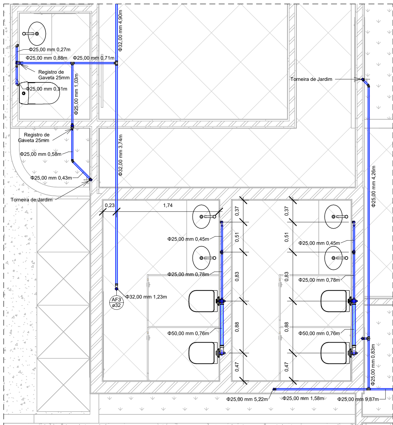
5 Detalhe 1 1 : 40
