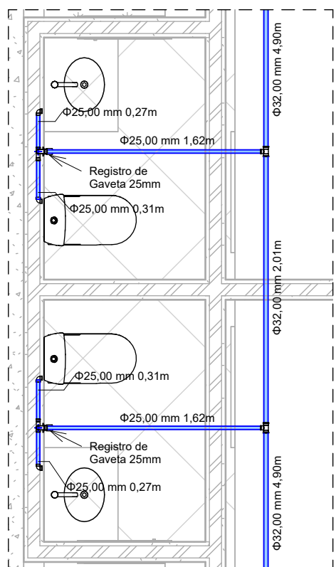
6 Detalhe 2 1 : 40
