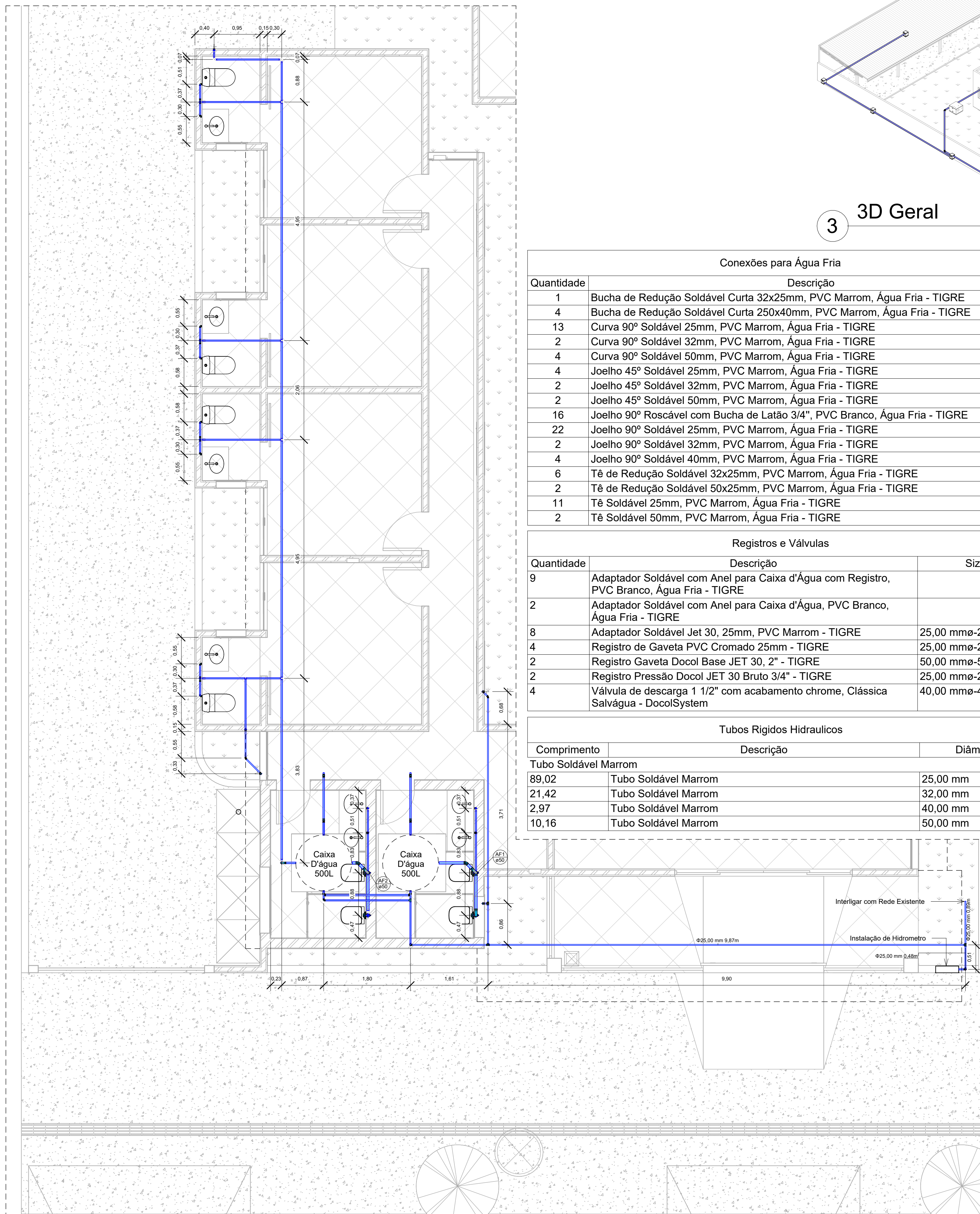
2 01 - Planta Hidraulica 1 : 50
