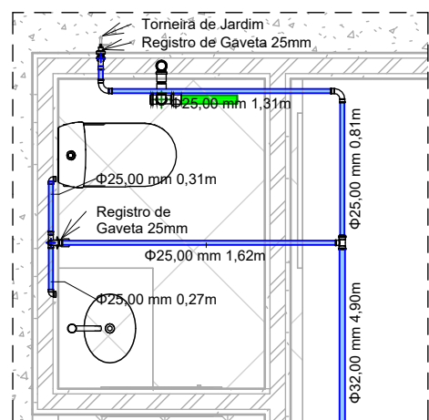
7 Detalhe 3 1 : 40
