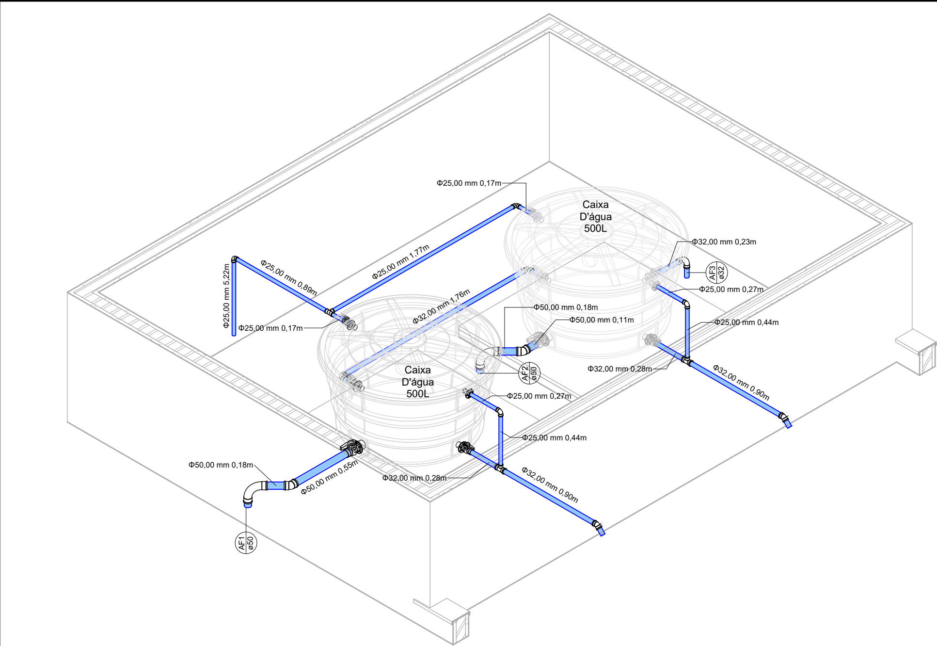
1 3D Detalhe Hidraulico 1
