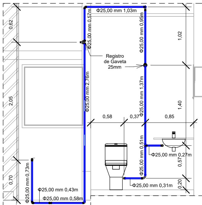
8 Detalhe 4 1 : 40
