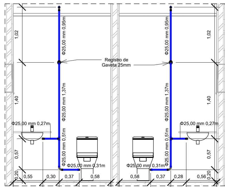
9 Detalhe 5 1 : 40
